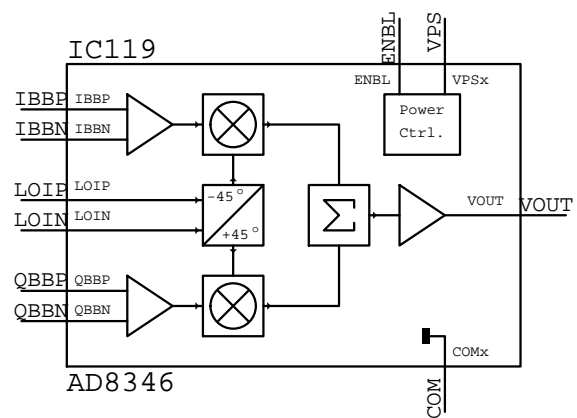
AD8346
