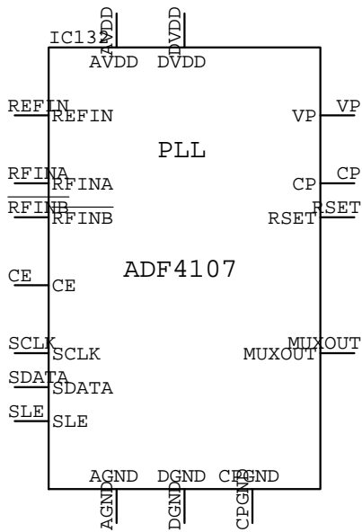
ADF4107
