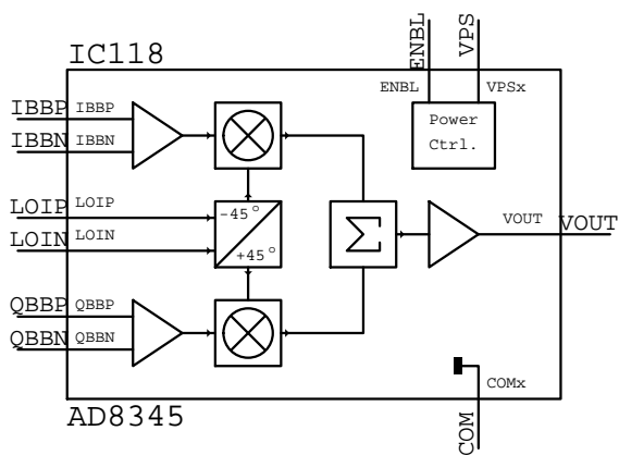
AD8345
