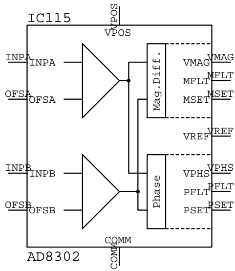
AD8302
