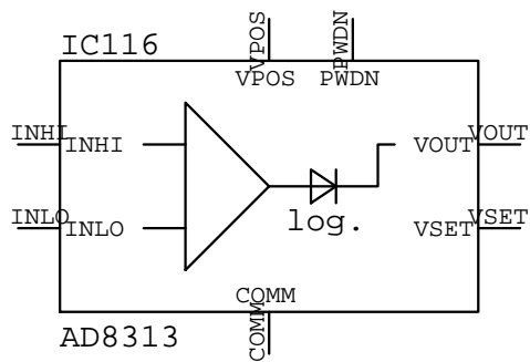
AD8313
