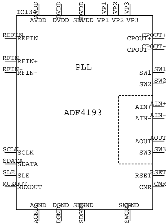
ADF4193
